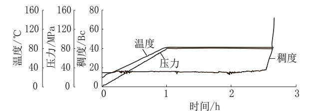
图2 尾浆稠化曲线
