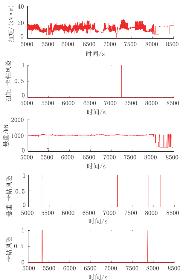
图5 WY-XX井卡钻故障预警结果
