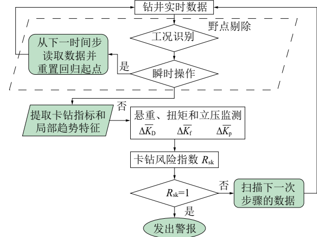
图 2 基于参数变化趋势异常诊断的卡钻实时预警流程
