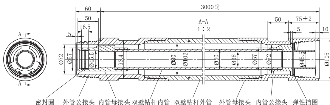
图1 双壁钻杆结构示意
