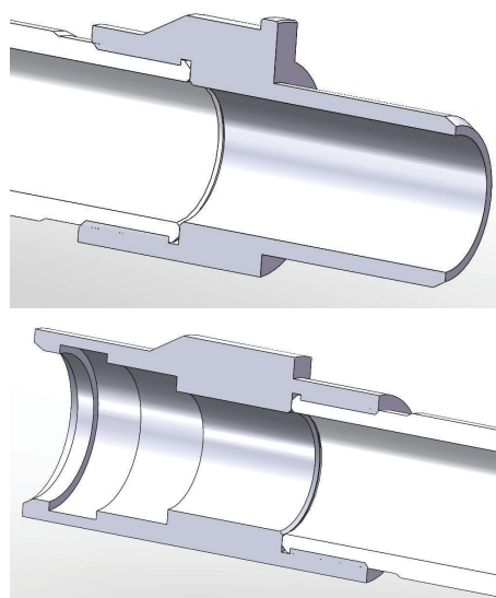
图3 双壁钻杆内管与内管公、母接头间的连接
