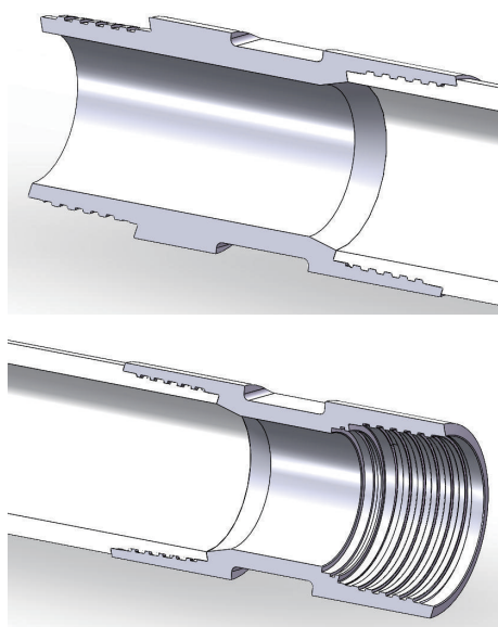
图2 双壁钻杆外管与外管公、母接头间的连接
