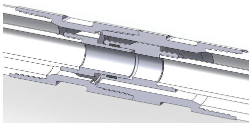
图5 两根独立的双壁钻杆总成间的连接
