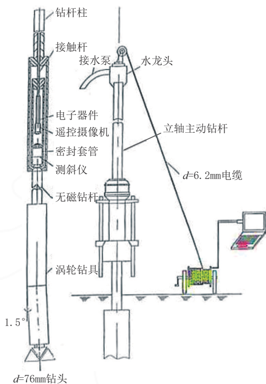
图8 小尺寸涡轮钻具钻进地质勘探定向孔用的设备 [12]
