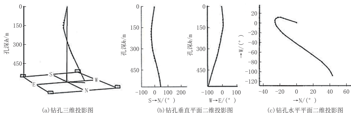
图11 钻孔剖面图
