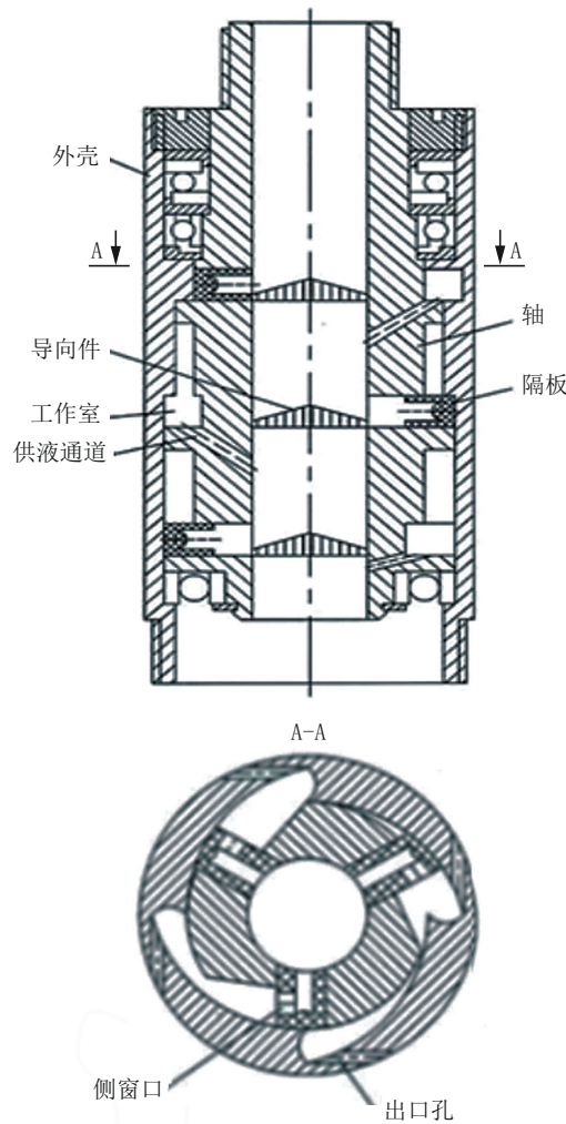
图3 3ГД-70型小尺寸涡轮钻具 Fig.3 Small-sized turbo drill 3ГД-70
