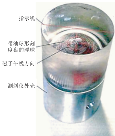
图9 导航系统中的 МИР-4 型多点测斜仪
