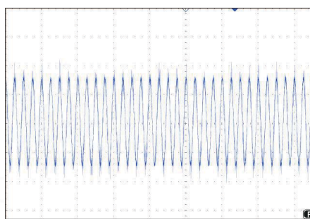
峰峰值 832mV 频率 40.19Hz 占空比 49.84% 最小值 -56.0mV 最大值 776mV
