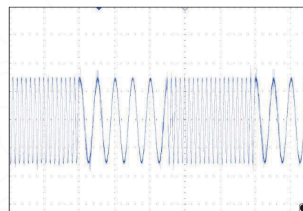
峰峰值 760mV 频率 2.365kHz 占空比 96.85% 最小值 8.00mV 最大值 768mV
