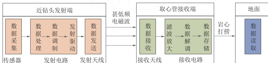
图2 信号传输流程
