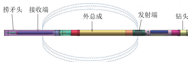
图1 系统整体方案示意
