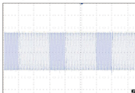
峰峰值 760mV 频率 168.1Hz 占空比 99.76% 最小值 8.00mV 最大值 768mV
