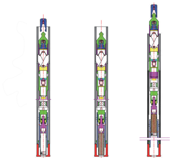
(a) 内总成送入 (b) 定向取心钻进 (c) 内总成回收
