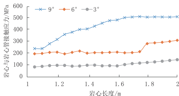
图10 不同造斜率条件下岩心与岩心管接触应力
