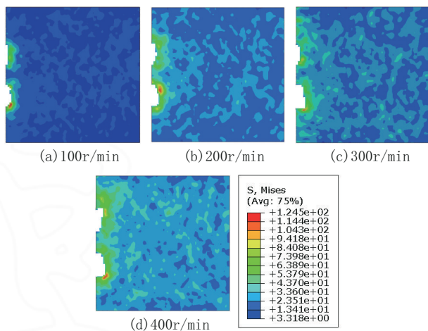
图9 不同转速下钻进岩层应力分布云图
