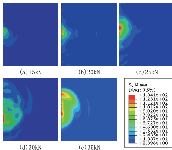
图 7 不同钻压下钻进岩层应力分布云图
