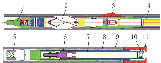
1—绳索打捞机构;2—弹卡定位机构;3—推靠导向机构;4—随钻测量存储探管;5—可提携式小口径大扭矩螺杆马达;6—偏心轴承组件;7—轻质高强取心管;8—传扭管;9—外管;10—岩心定向机构;11—定向取心钻头
