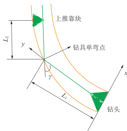
图3 定向钻进连续取心钻具造斜模型示意
