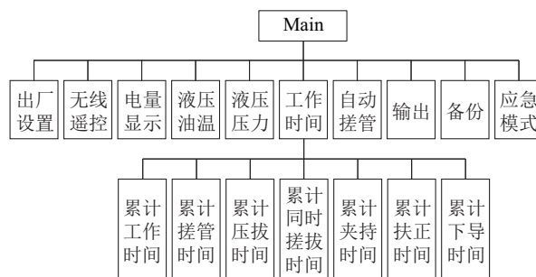
图7 PLC程序结构
