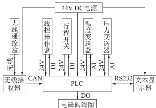
图4 供电及通信电路设计框图
