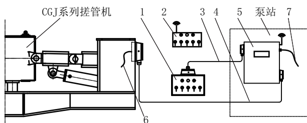
1—线控操作盒;2—无线遥控盒;3—线控电缆;4—钻机电缆;5—PLC电控箱;6—钻机电线束;7—泵站线束
