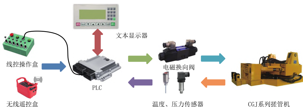
图2 电控系统拓扑图
