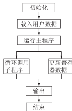
图8 PLC程序流程
