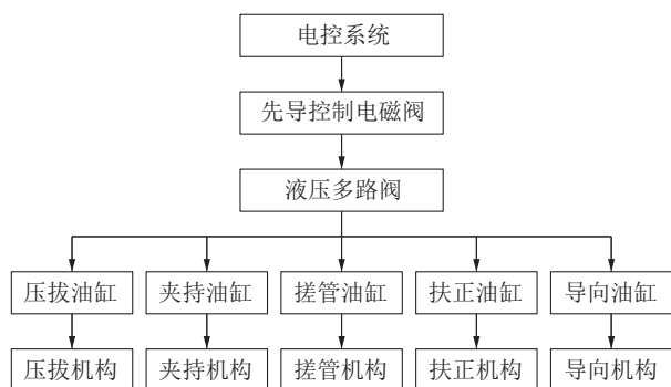
图1 搓管机系统架构
