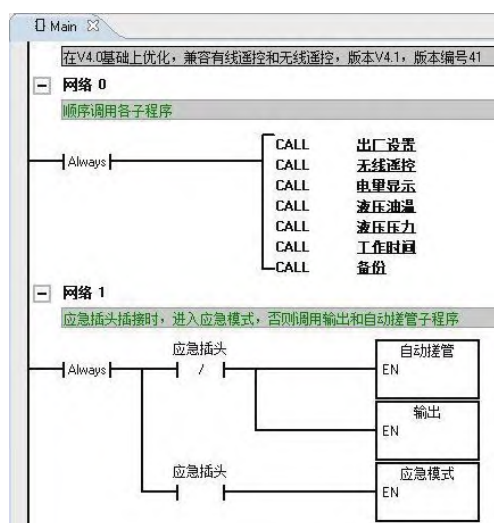
图9 PLC主程序
