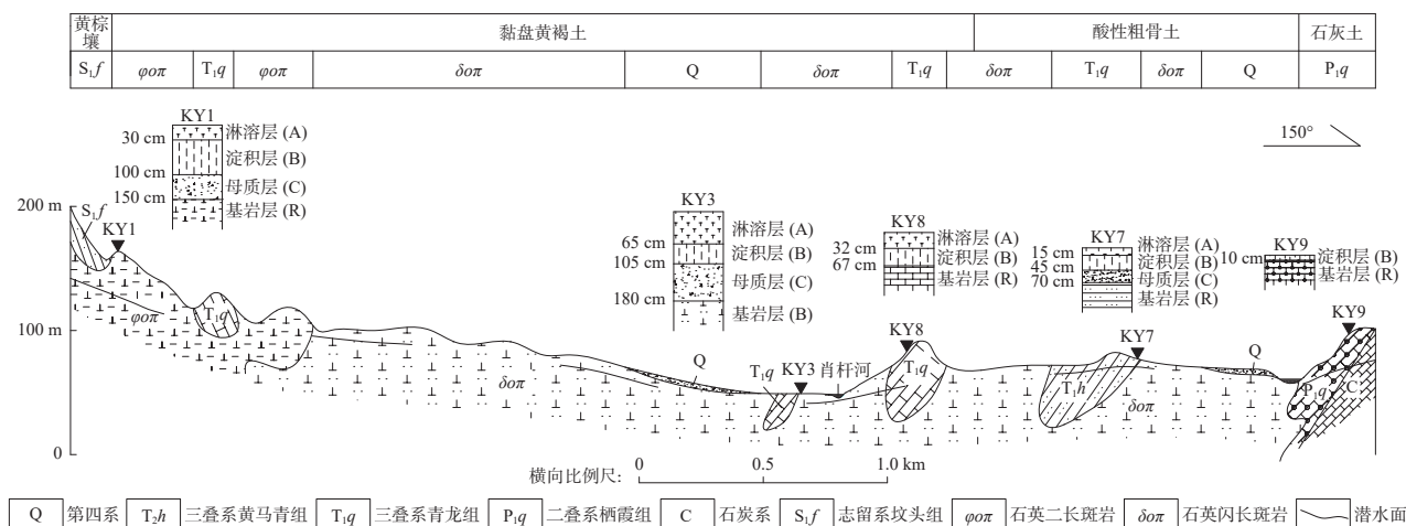
图2 研究区生态地质剖面图
