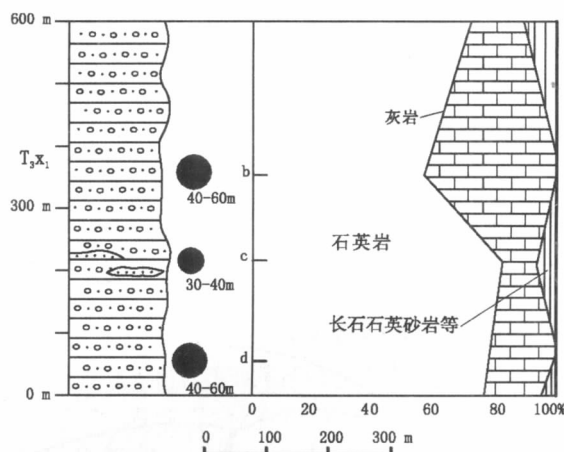
图 2 小河口组红石砬子磨拉石砾径及成分统计图 (据 1:20 万浑江市、集安幅, 1976, 修改)
