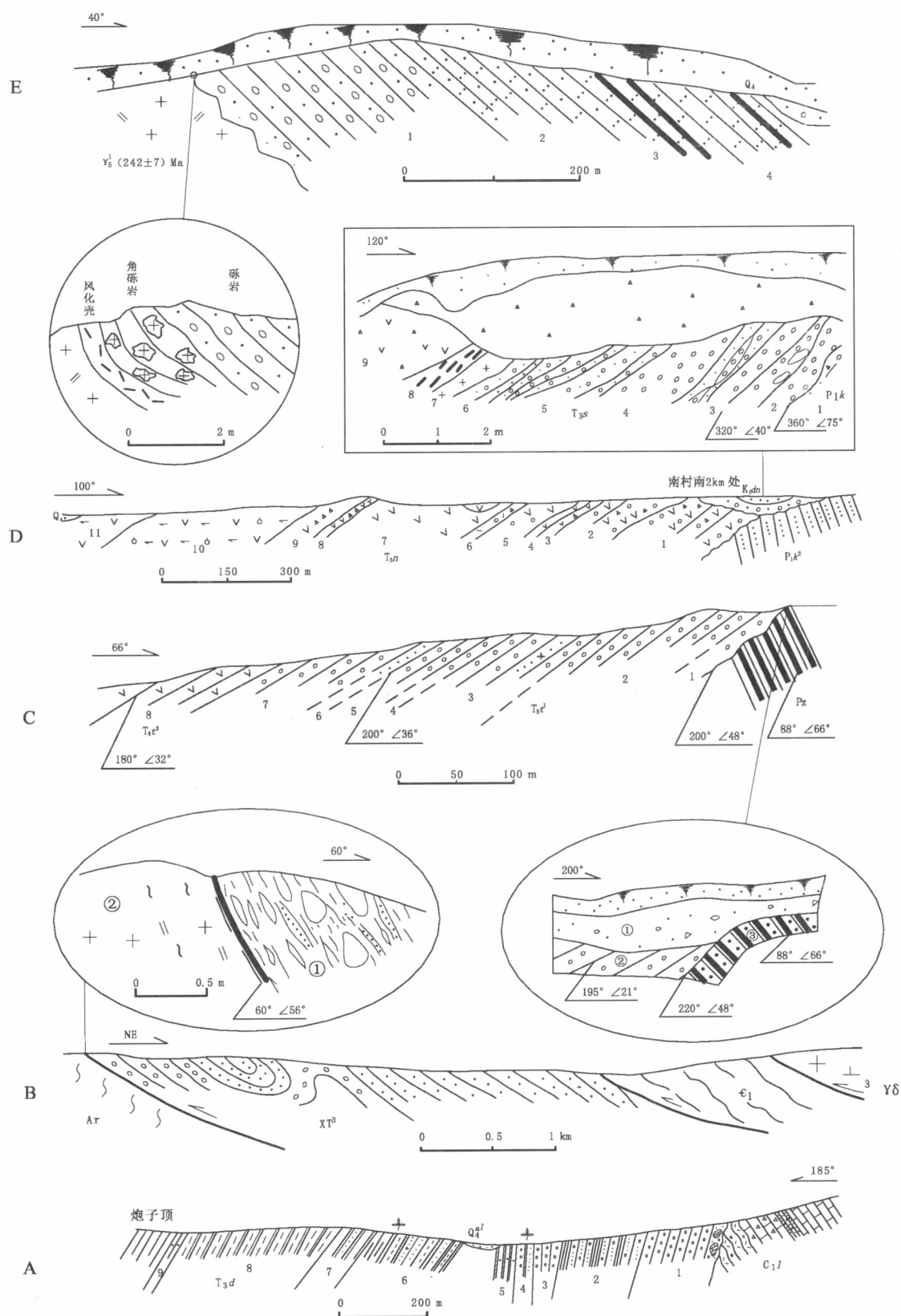
图1 吉林、黑龙江省三叠世地层底部磨拉石与下伏地层角度不整合实测剖面及素描图
