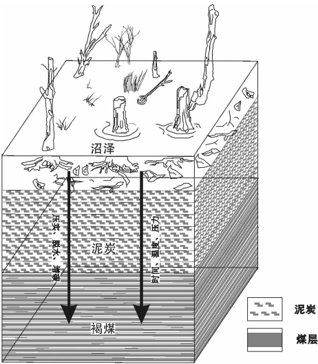
图 1 泥炭的形成和转化 Fig.1 Peat formation and transformation
