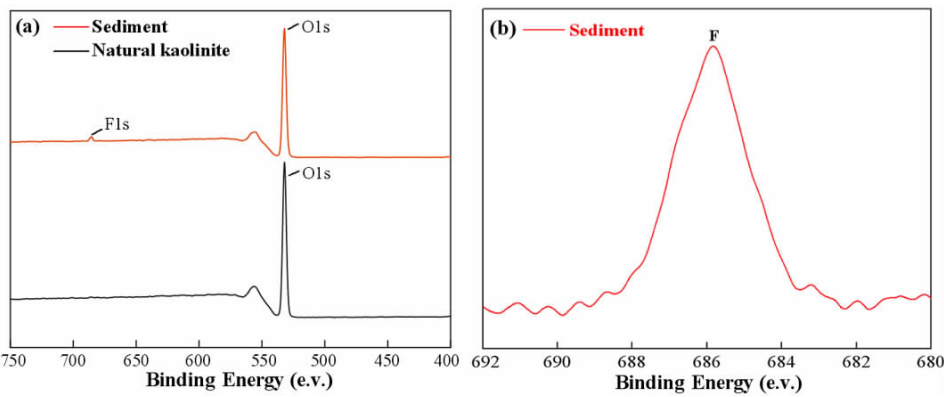
图 10 天然高岭石及除氟渣的 XPS 全谱(a), F1s 的 XPS 窄谱(b) Fig. 10 (a) XPS full spectrum of natural kaolinite and defluorinated residue, (b) XPS narrow spectrum of F1s
