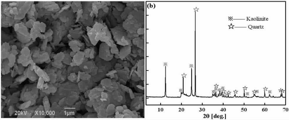
图 2 天然高岭石的 (a) SEM 图, (b) XRD 图 Fig. 2 (a) SEM and (b) XRD of natural kaolinite
