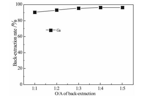
图12 相比对镓反萃取率的影响 Fig. 12 Effect of O/A on back-extraction rate of Ga
