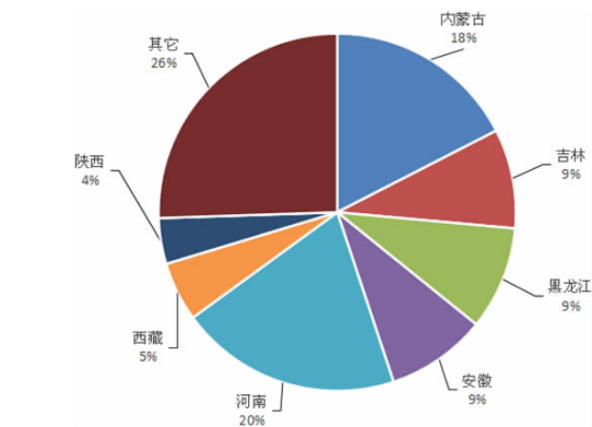
图 3 2017 年中国钼查明资源储量分布 Fig. 3 Distribution of molybdenum resources in China in 2017
