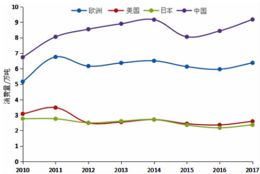
图 7 2010—2017 年世界钼消费变化趋势 Fig. 7 Variation trends of molybdenum consumption in the world from 2010 to 2017 数据来源:wind 资讯。
