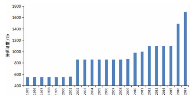
图 1 全球钼矿资源储量变化趋势 Fig. 1 Variation trends of global molybdenum reserves
