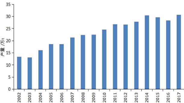
图 4 2002—2017 年全球矿山钼产量变化趋势 Fig. 4 Variation trends of global molybdenum production from 2002 to 2017
