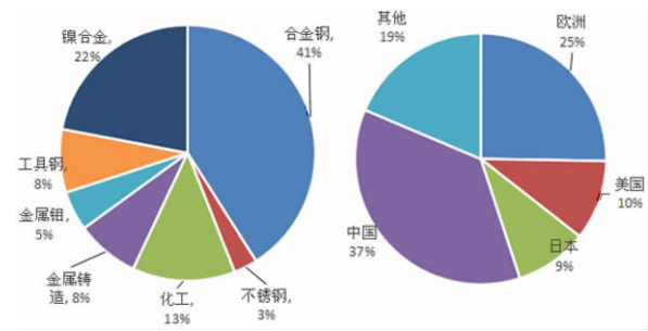
图 8 全球钼终端消费(左)和区域消费(右)结构图 Fig. 8 Molybdenum terminal consumption( Left) and consumption structure( Right) 资料来源:根据公开资料整理。
