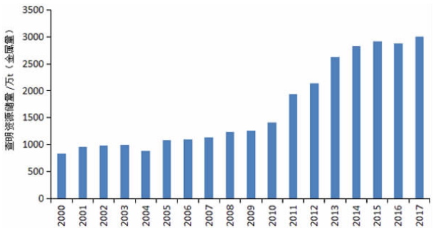
图 2 2000—2017 年中国钼查明资源储量变化情况图 Fig. 2 Variation of molybdenum identified reserves in China from 2000 to 2017
