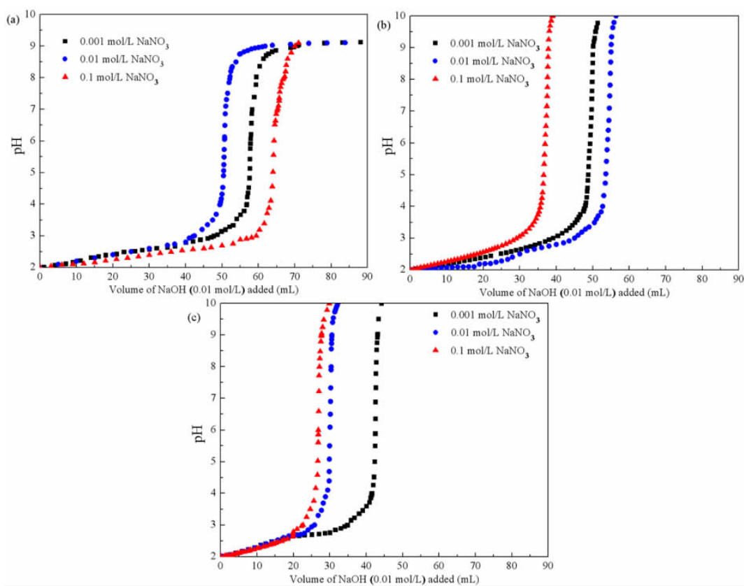
图 2 \text{S}^0 (a)、 \text{Fe}^{2+} (b)、 \text{FeS}_2 (c) 培养的 A. ferrooxidans 不同离子强度酸碱滴定曲线 Fig. 2 Potentiometric titration data of A. ferrooxidans cultured with \text{S}^0 (a), \text{Fe}^{2+} (b) and \text{FeS}_2 (c) at different ionic strengths
