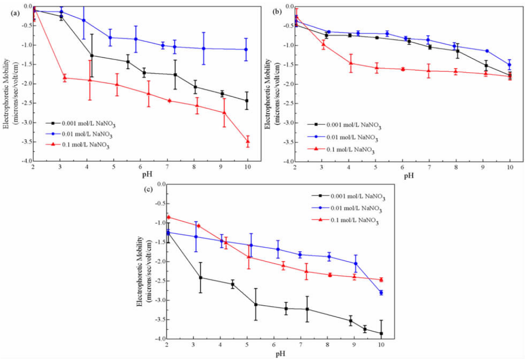
图 4 S^0 (a)、 Fe^{2+} (b)、 FeS_2 (c) 培养的 A. ferrooxidans 不同离子强度电泳迁移率 Fig. 4 Electrophoretic mobility data for A. ferrooxidans cultured with S^0 (a), Fe^{2+} (b) and FeS_2 (c) at different ionic strengths
