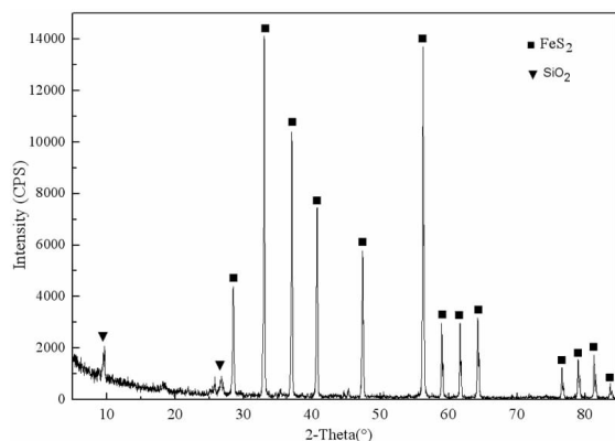
图 1 黄铁矿 X 射线衍射图
