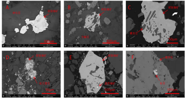
A: 钾长石包裹铌钽铀矿;B: 方解石包裹铌钽铀矿;C: 铌钽铀矿包裹磷灰石;D: 铌钽铀矿与铅贝塔石共生;E: 铌钽铀矿包裹晶质铀矿;F: 褐帘石包裹钽石
