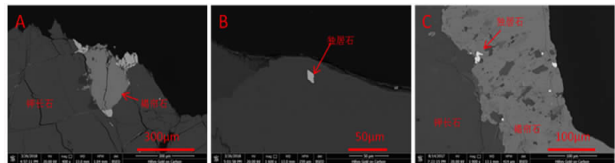
图 4 稀土矿物照片 Fig. 4 rare earth elements minerals
