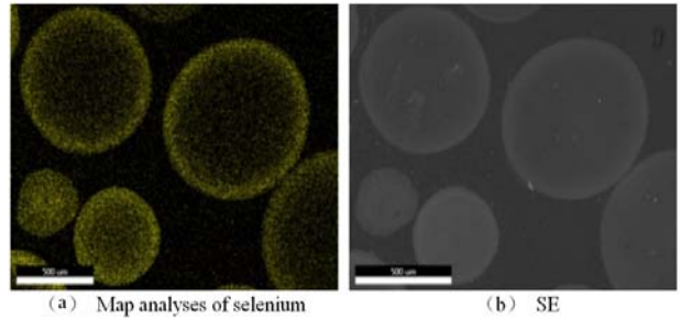
图 6 饱和树脂电子探针分析
