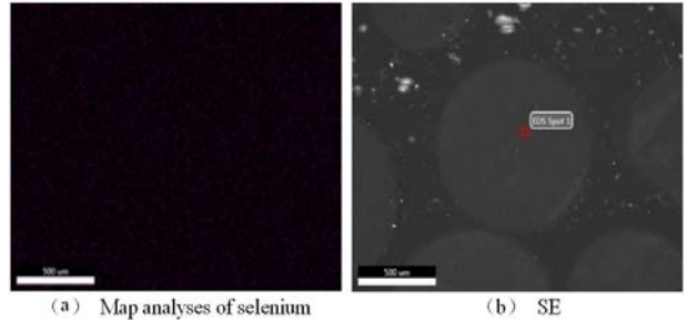
图 5 新树脂电子探针分析
