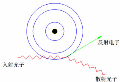
图 1 电子对效应示意图
