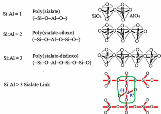
图1 碱地质聚合物结构
