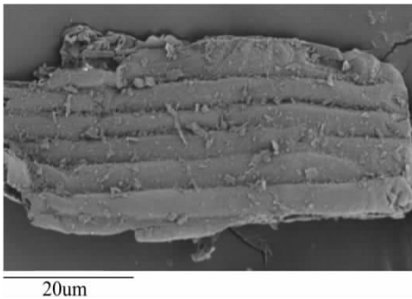
图 1 椰壳活性炭的电镜扫描图 Fig. 1 SEM images of CSCC
