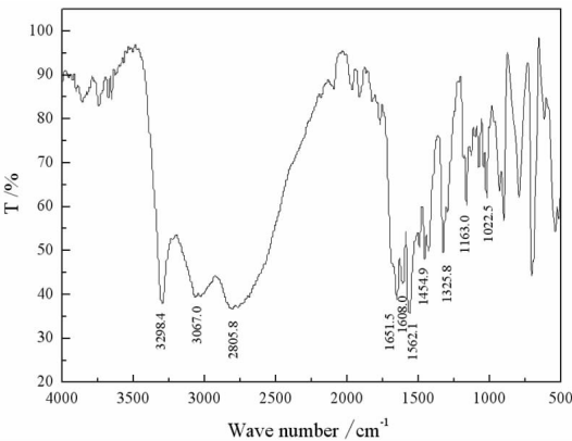
图 8 GYB 药剂的红外光谱图 Fig. 8 The infrared spectroscopy chart of GYB reagent
