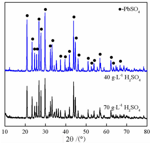
图 5 不同硫酸浓度下浸出渣的 XRD 谱 Fig. 5 XRD patterns of the leaching residue at different \text{H}_2\text{SO}_4 concentration
