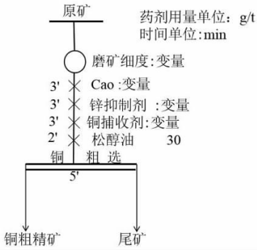
图 2 铜粗选试验流程 Fig. 2 Experimental flowsheet of copper roughing
