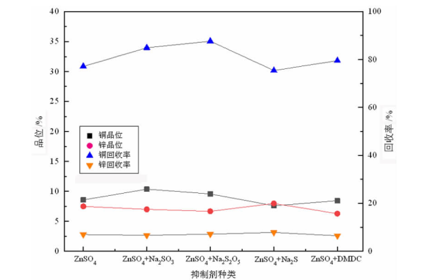
图5 锌抑制剂种类试验结果 Fig. 5 Results of zinc depressant types tests
