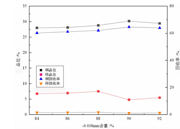
图 7 再磨细度试验结果 Fig. 7 Results of regrinding fineness test
