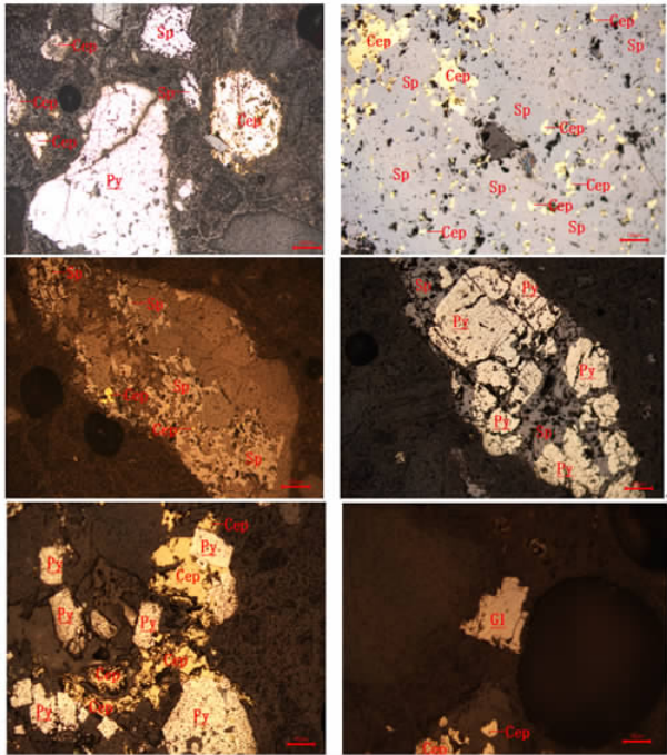
图 1 原矿显微镜下观察图 Fig. 1 Observation diagram of raw ore under microscope
