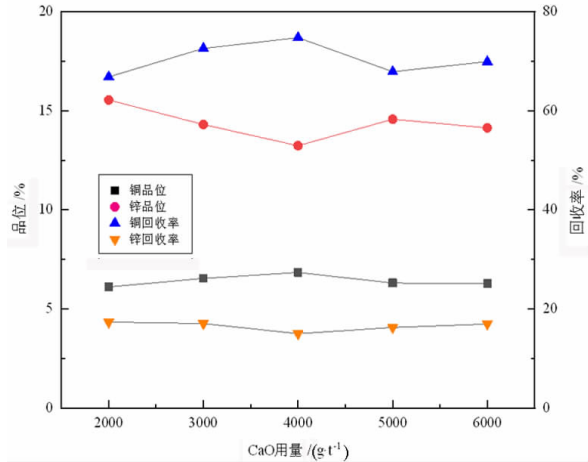
图 4 石灰用量试验结果 Fig. 4 Results of CaO dosage tests
