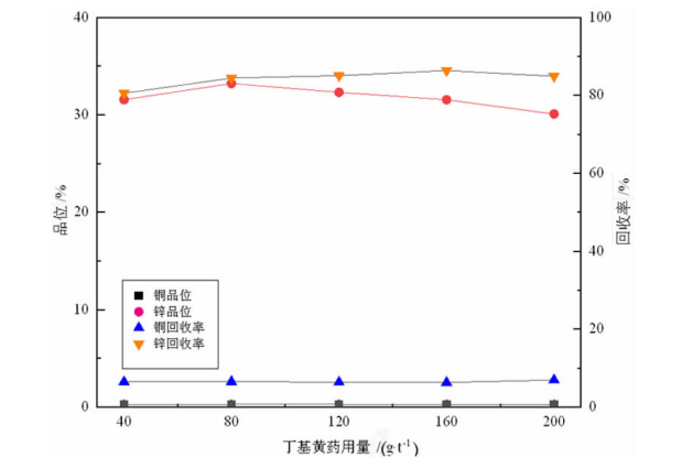
图11 丁基黄药用量试验结果 Fig. 11 Results of Isobutyl xanthate dosage tests
