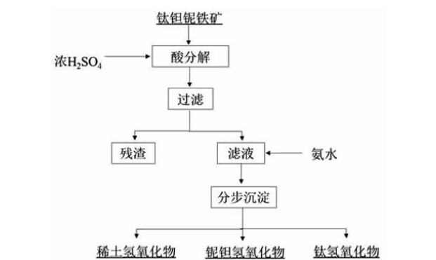
图 4 硫酸法分解工艺流程 Fig. 4 Process flow of sulfuric acid decomposition
