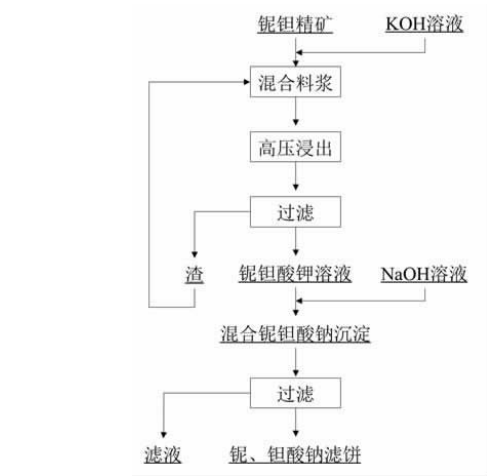
图 6 碱性水热法工艺流程 Fig. 6 Flow chart of alkaline hydrothermal process
