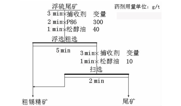
图 4 浮锡捕收剂种类试验流程 Fig. 4 Test flowsheet of collector type
