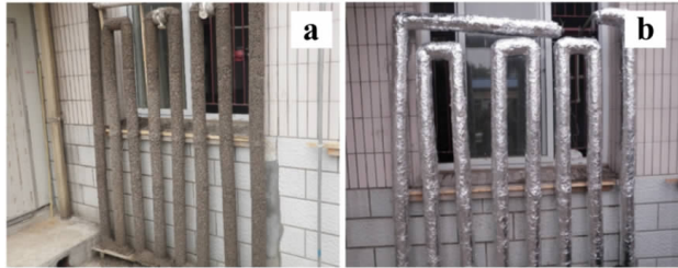
图5 管道保温层水泥基保温砂浆的施工(a. 保温层的施工;b. 防水层的施工)
