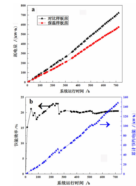
图4 样板房能耗与保温样板房节电量、节能效率与运行时间的关系(a.耗电量;b.节约电量、节能效率)
