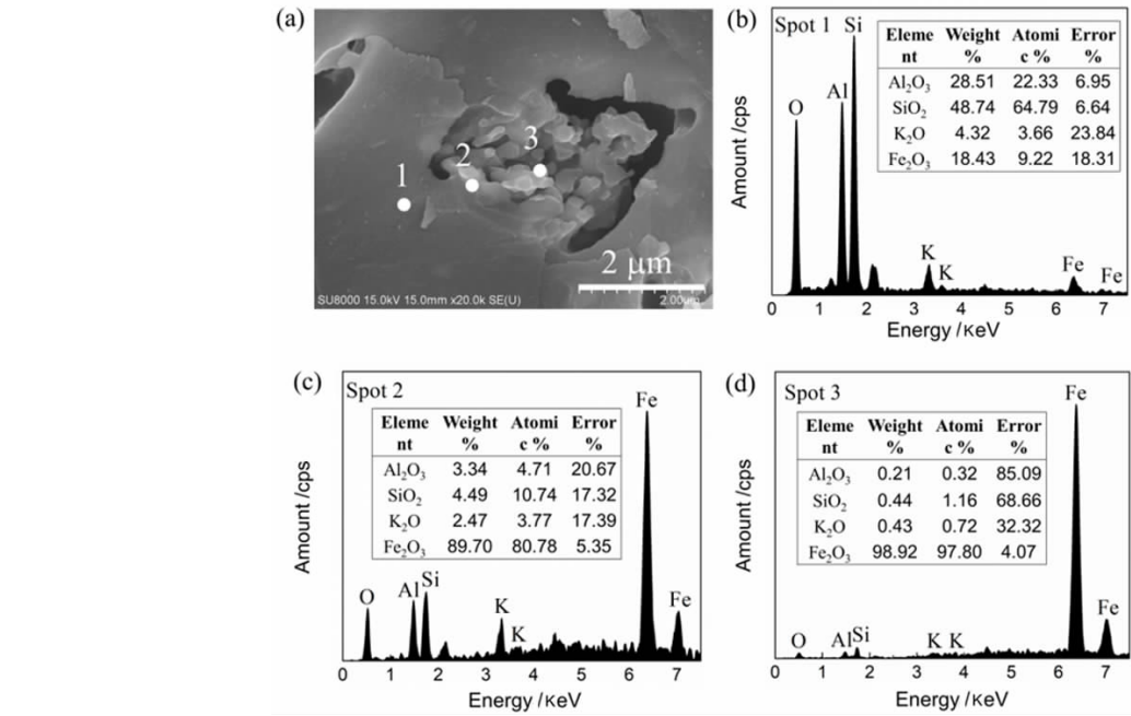
图 6 清水泥孔道的 EDS 能谱图及孔道周围的化学成分分析结果
