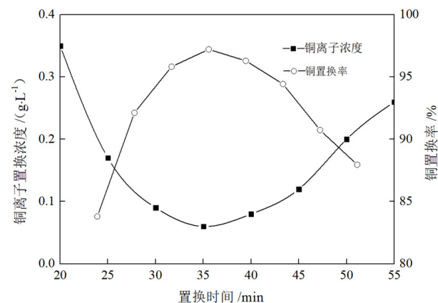
图9 置换时间试验结果
