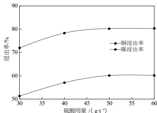
图5 硫酸用量试验结果
