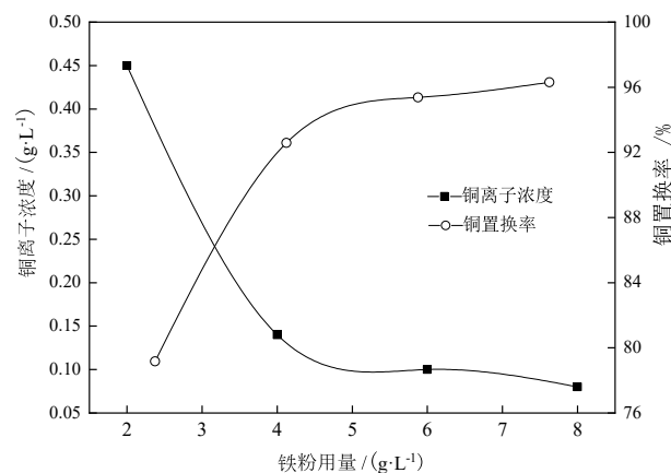
图8 铁粉用量试验结果
