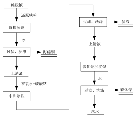
图7 铜镍分离原则工艺流程
