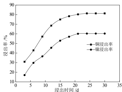
图6 浸出时间试验结果
