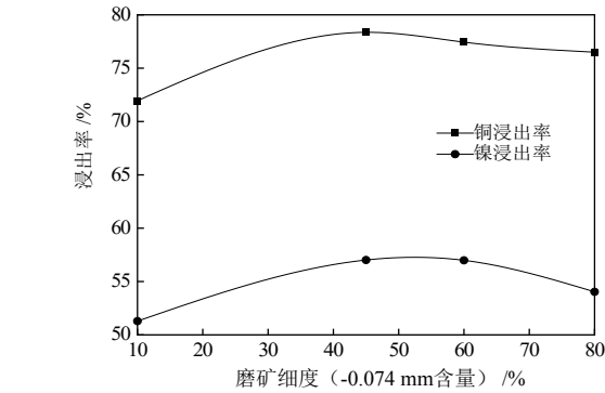
图 4 磨矿细度试验结果 Fig. 4 Results of grinding fineness test
