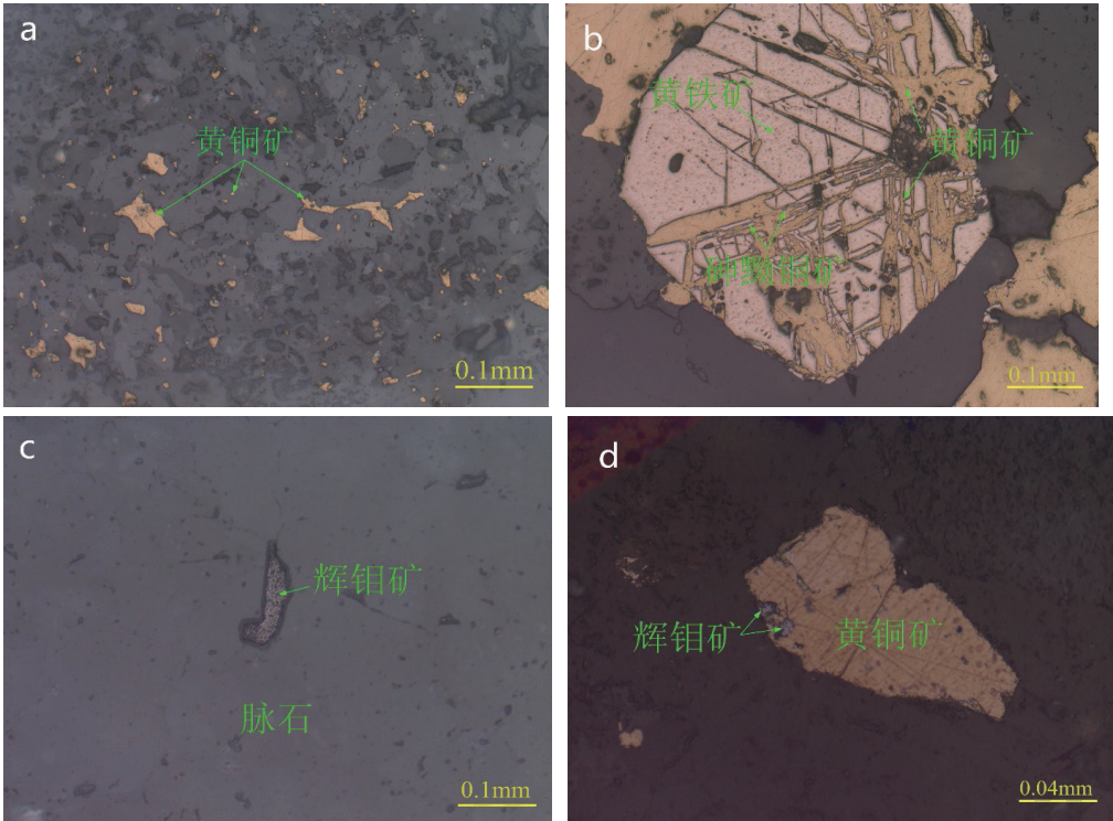
图 1 原矿显微镜下观察图 Fig. 1 Observation diagram of raw ore under microscope
