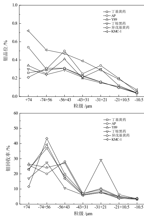
图 6 不同捕收剂对各粒级钼品位及钼分布的影响
