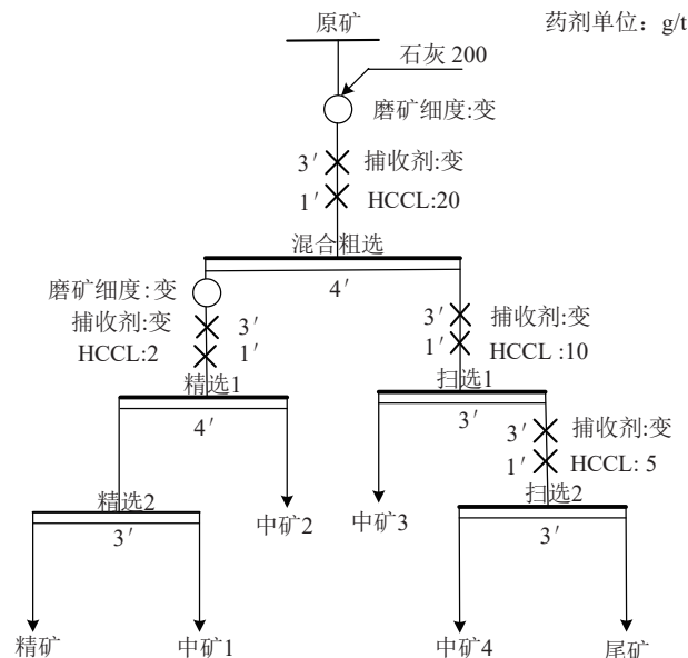
图 2 铜钼混合试验流程
