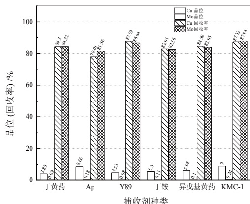
图 4 捕收剂种类试验结果
