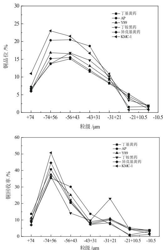
图 5 不同捕收剂对各粒级铜品位及铜分布的影响
