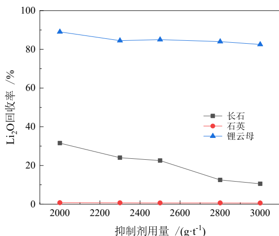
图5 六偏磷酸钠用量对单矿物浮选的影响
