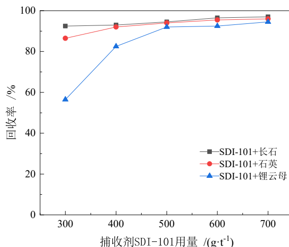
图3 捕收剂 SDI-101 用量对单矿物浮选的影响
