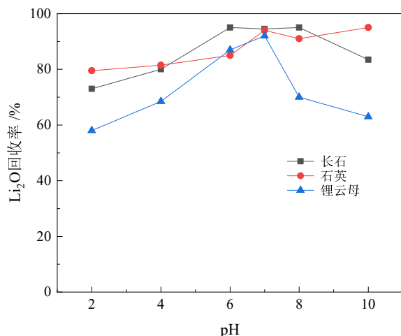
图4 矿浆 pH 值对单矿物浮选的影响
