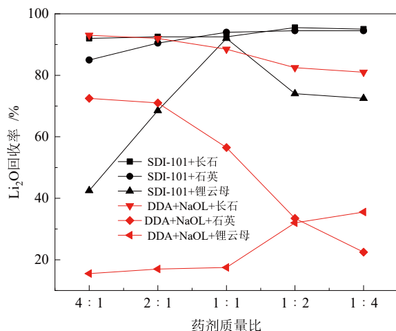
图2 药剂质量比对单矿物浮选的影响
