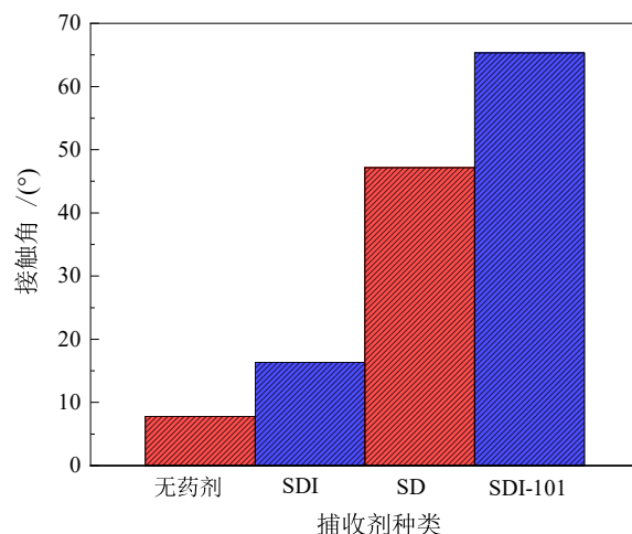
图6 几种药剂作用前后锂云母接触角变化
