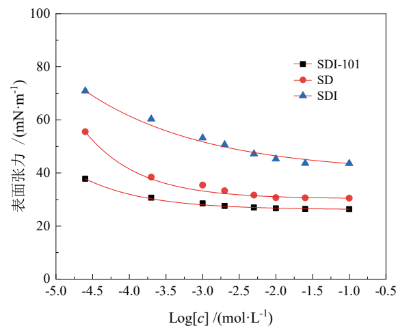
图7 几种捕收剂表面张力测量结果
