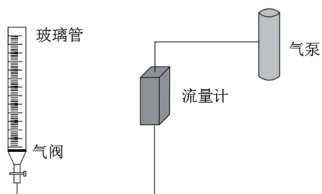
图1 泡沫性能测试装置
