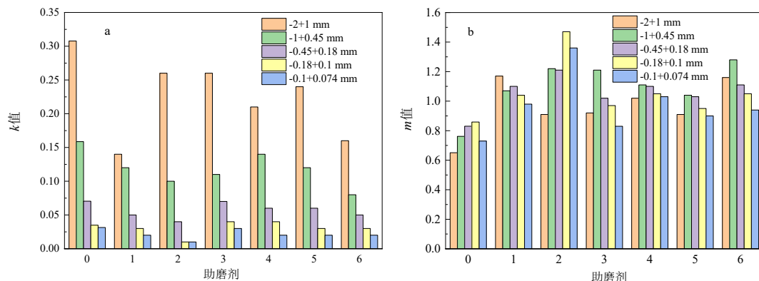
图6 助磨剂对石英粉磨 m 阶磨矿动力学模型参数 k 和 m 的影响
