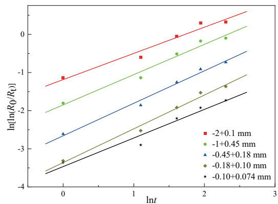
图3 不同粒级的 \ln[\ln(R_0/R_t)] 与 \ln t 的关系曲线
