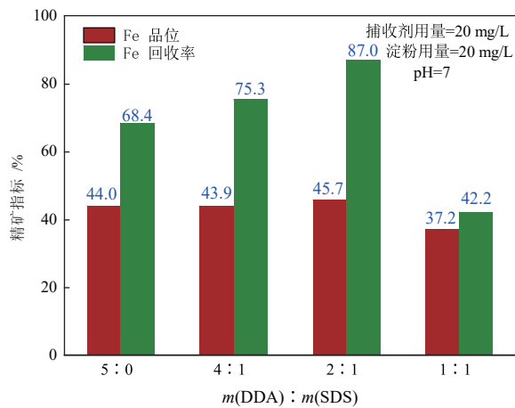
图9 人工混合矿物浮选结果
