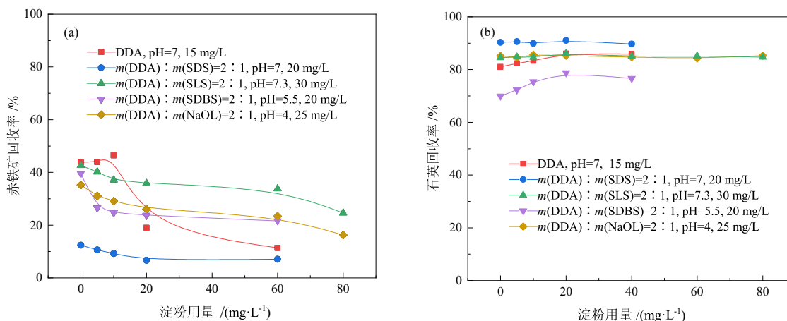
图 8 不同捕收剂体系中淀粉用量对赤铁矿(a)和石英(b)回收率的影响
