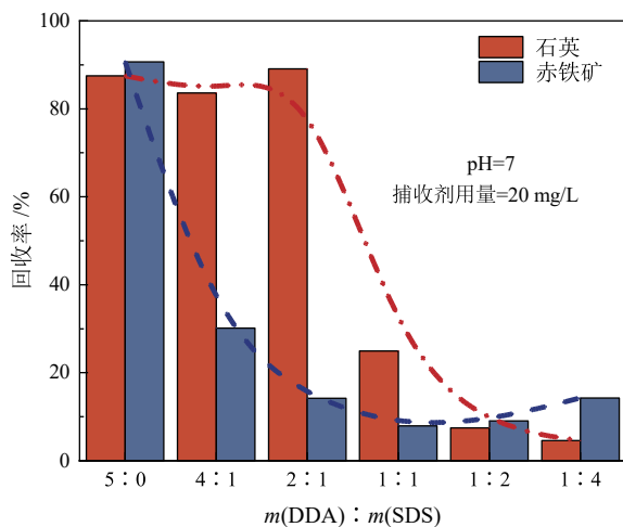
图4 十二胺与十二烷基磺酸钠的质量比对赤铁矿和石英回收率的影响
