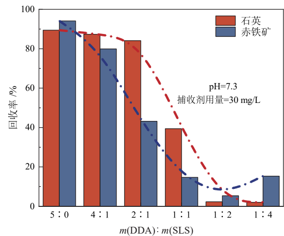
图5 十二胺与十二烷基硫酸钠的质量比对赤铁矿和石英回收率的影响
