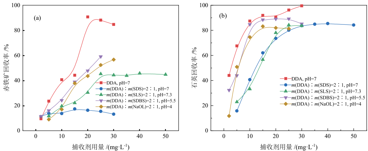
图3 不同捕收剂体系中捕收剂用量对赤铁矿(a)和石英(b)回收率的影响
