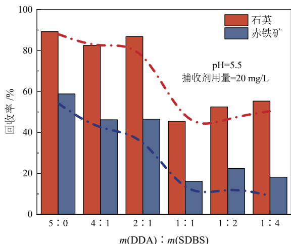
图 6 十二胺与十二烷基苯磺酸钠的质量比对赤铁矿和石英回收率的影响
