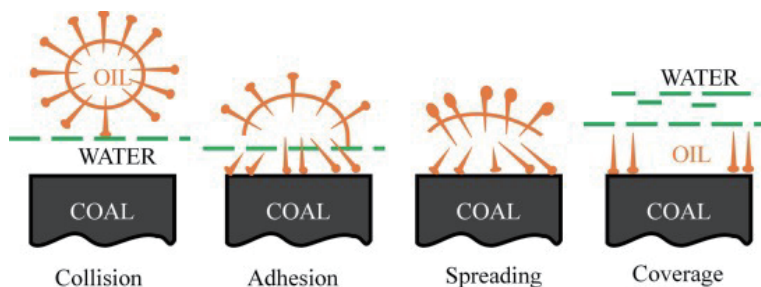
图5 非离子表面活性剂乳化药剂液滴在煤/水界面的润湿过程示意图 [45]
