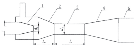
1—喷嘴;2—吸气室;3—喉管;4—扩散管;5—尾管
