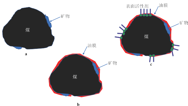
图6 药剂与煤的作用机理 [32] (a—未加捕收剂的煤粒;b—加油类捕收剂的煤粒;c—加乳化药剂的煤粒)
