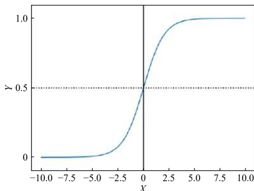
图 2 Sigmoid 函数
