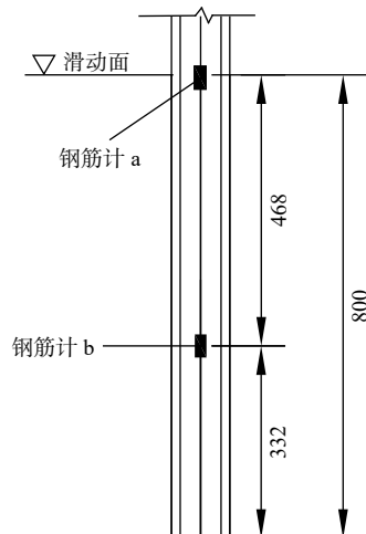
图 3 钢筋计布置示意图 (单位: mm)
