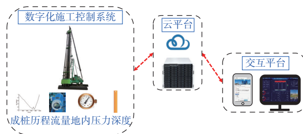
图1 数字化搅拌桩施工云平台构成
