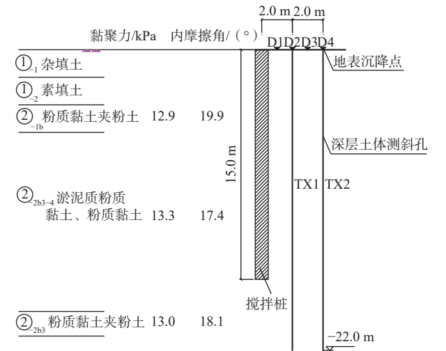
图 5 监测点剖面布置图 Fig. 5 Profile layout of the monitoring points
