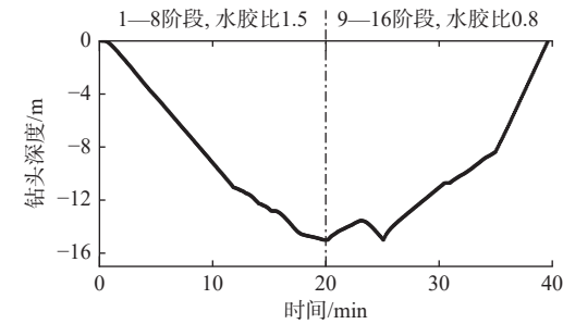
图 6 成桩分段水胶比控制 Fig. 6 Water binder ratio control of the construction section
