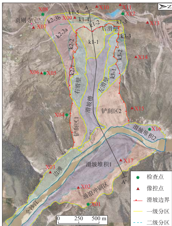
图 3 白格滑坡监测分区 (2021 年 9 月 28 日正射影像)
