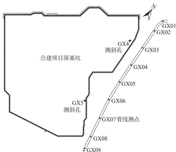
图5 测点与基坑平面位置关系
