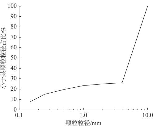
图2 颗粒级配
