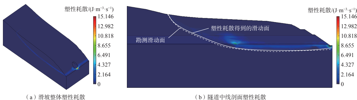
图 10 未处理时的滑坡塑性耗散
