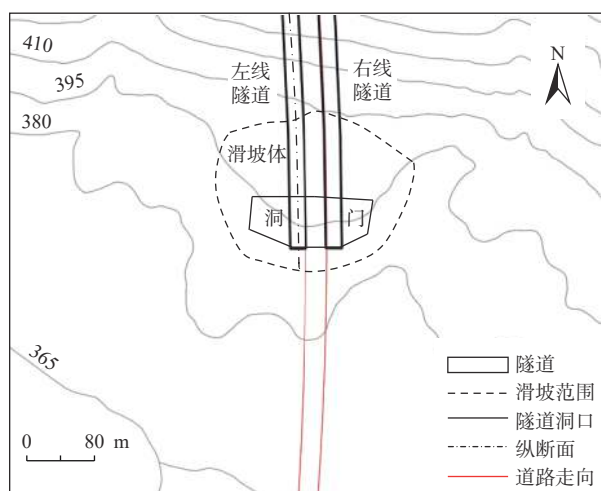
图1 场地平面图
