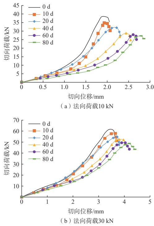
图 4 切向加载位移-荷载曲线 Fig. 4 Tangential loading displacement-load curve
