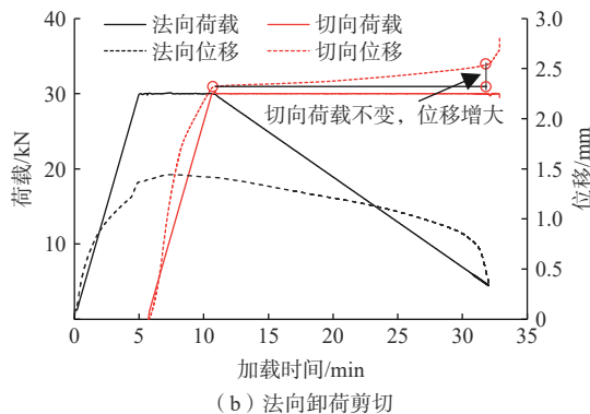
图 3 剪切试验过程中荷载/位移-时间曲线
