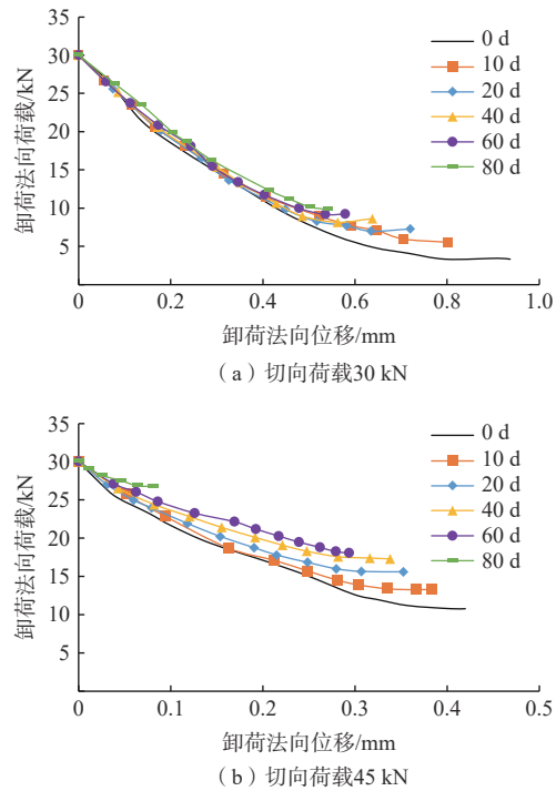
图 5 法向卸荷阶段荷载-位移曲线 Fig. 5 Load-displacement curve at normal unloading stage
