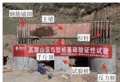
(c) 竖向静载试验装置
