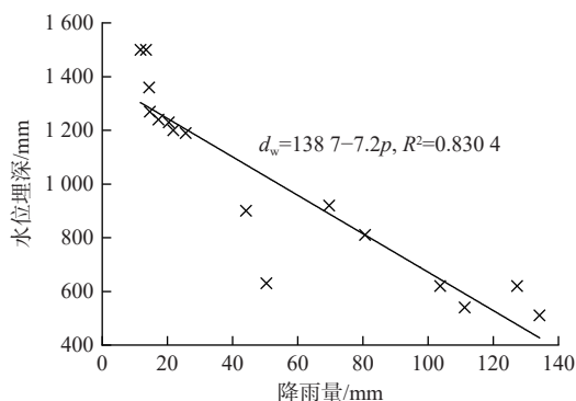
图 7 地下水埋深随日降雨量变化 Fig. 7 Groundwater depth vs. daily precipitation
