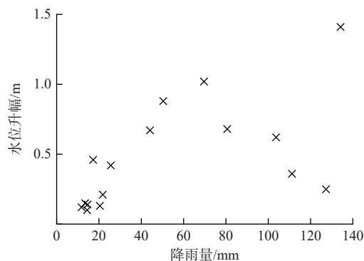
图 6 地下水位升幅随日降雨量的关系变化 Fig. 6 Groundwater level rising vs. daily precipitation
