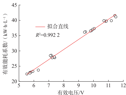
图 7 有效能耗系数与有效电压的关系
