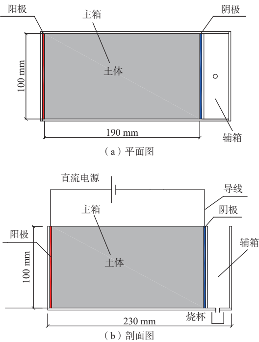
图 1 主体装置示意图 Fig. 1 Main device diagram
