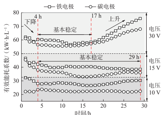
图 6 电渗中有效能耗系数的发展
