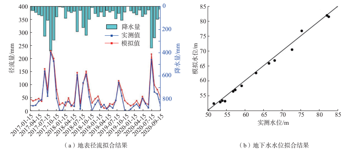
图 5 耦合模型地表径流量和地下水水位拟合结果 Fig. 5 Surface runoff and groundwater level in the coupling model
