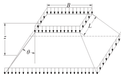
图2 钢架-土工材料系统应力扩散示意图
