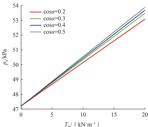
图 7 p_u 与 T_m 间的关系
