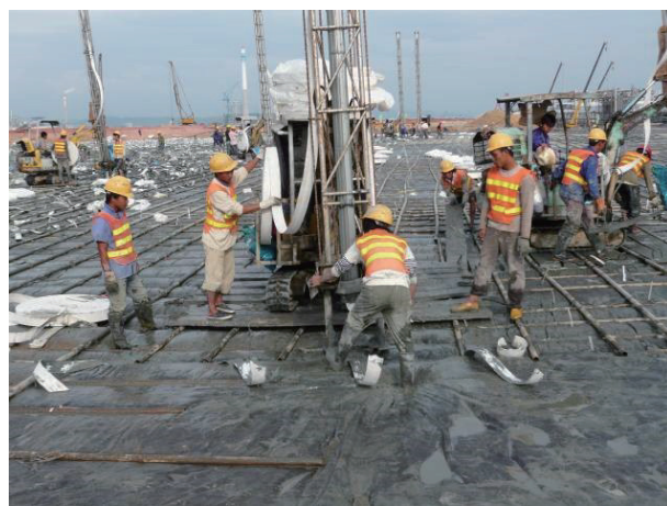
图 6 插板施工现场
