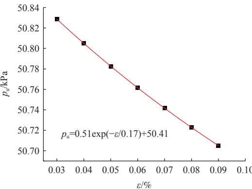
图 8 p_u 与土工材料 \varepsilon 间的关系
