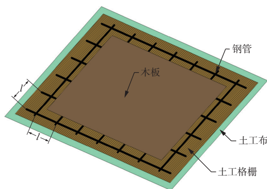
图1 钢架-土工材料系统
