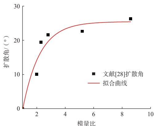
图9 应力扩散角与变形模量比间的关系
