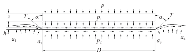
图 4 土工材料的受力情况示意图
