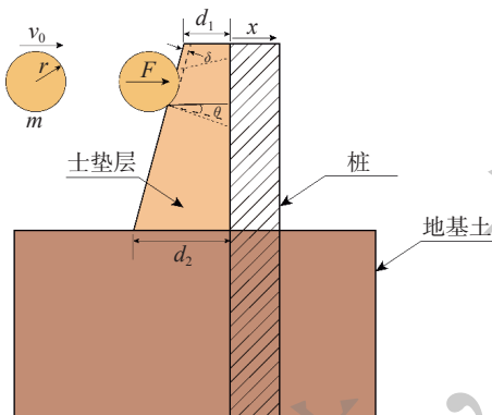
图 2 落石冲击作用下悬臂桩受力分析计算示意图( \theta 一般取 45^\circ-\varphi_k/2 , \varphi_k 为垫层材料内摩擦角)
