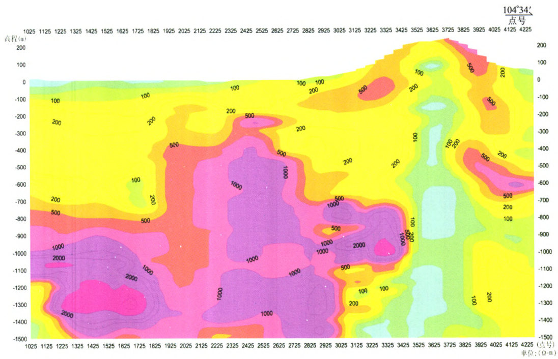
图 3 白象山铁矿 11 线 CSAMT 勘查电阻率断面图 Fig. 3 CSAMT prospecting resistivity section of exploration line 11 in the Baixiangshan iron deposit
