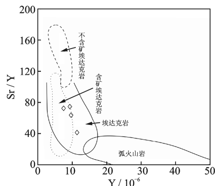
图 9 白马山小岩体 Sr/Y-Y 图解(底图据文献[27])
