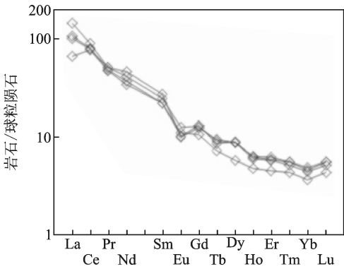
图 4 白马山岩体稀土元素球粒陨石标准化配分曲线图 (球粒陨石数据引自文献[3]) Fig.4 Chondrite-normalized REE patterns for the Baimashan rock mass
