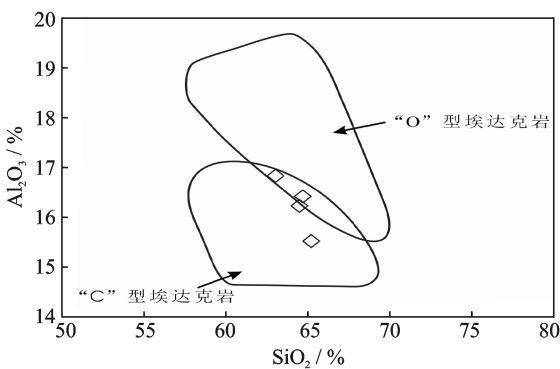
图 3 白马山岩体 SiO 2 -Al 2 O 3 图解(底图据文献[2]) Fig.3 SiO 2 vs. Al 2 O 3 diagram of the Baimashan rock mass
