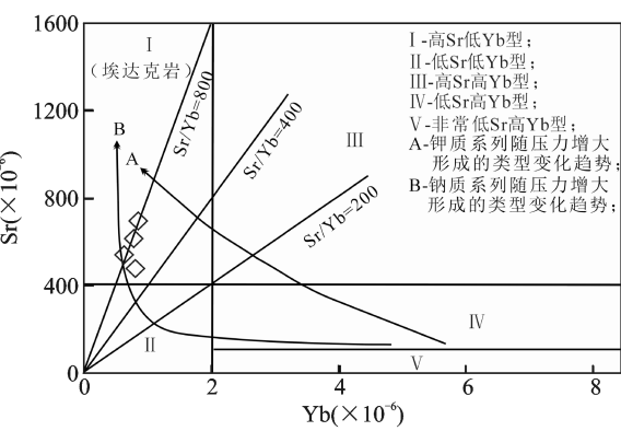
图 5 白马山岩体 Sr-Yb 图解(底图据文献[2]) Fig.5 Sr vs. Yb diagram of the Baimashan rock mass
