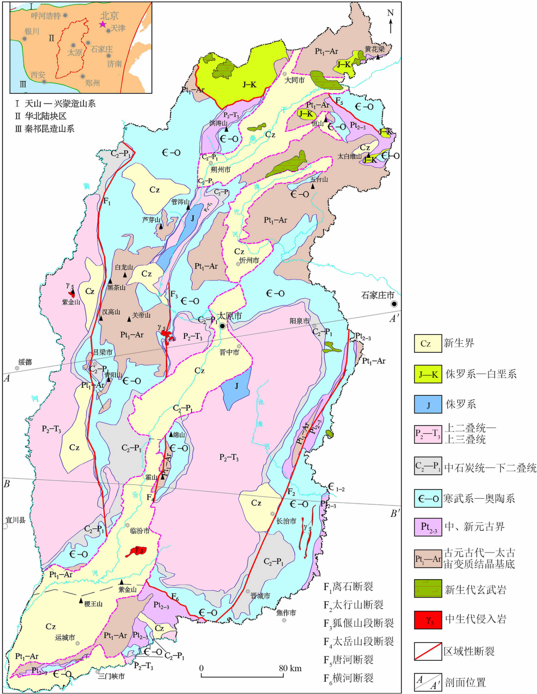
图 1 山西省地质简图
