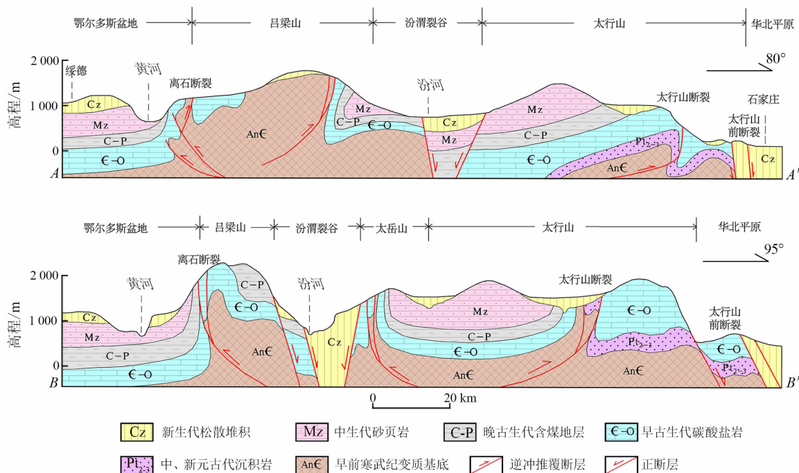
图2 山西隆起区横向构造剖面示意图
