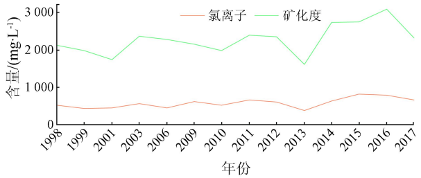
图 8 广饶县石村监测点矿化度和氯离子含量变化曲线
