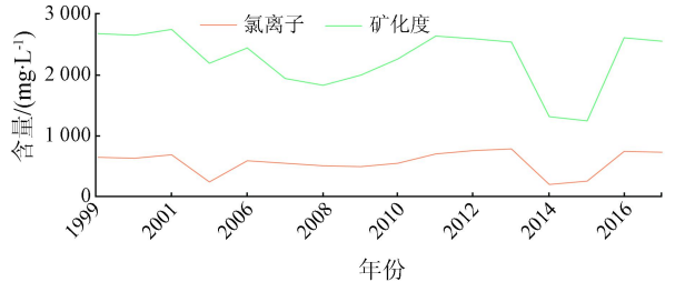
图 10 广饶县肖家村监测点矿化度和氯离子含量变化曲线
