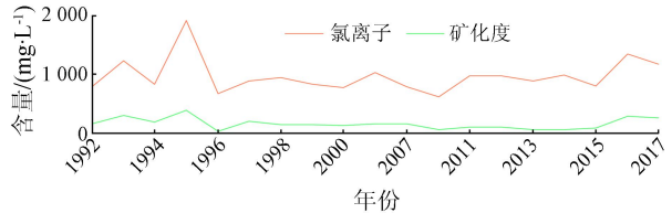
图 9 广饶县甄庙村监测点矿化度和氯离子含量变化曲线
