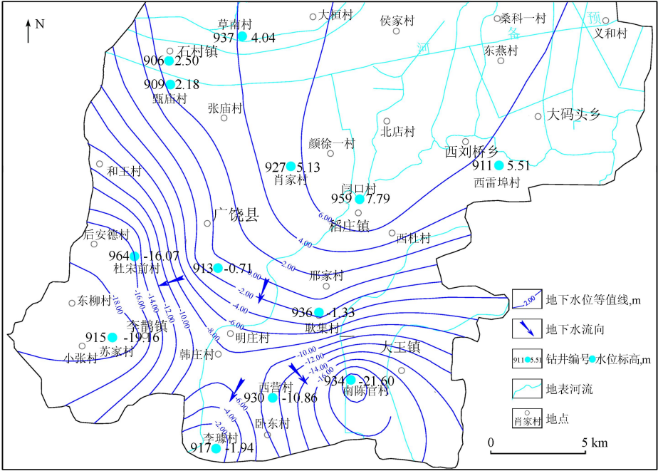
图3 2016 年 9 月广饶县南部浅层地下水降落漏斗
